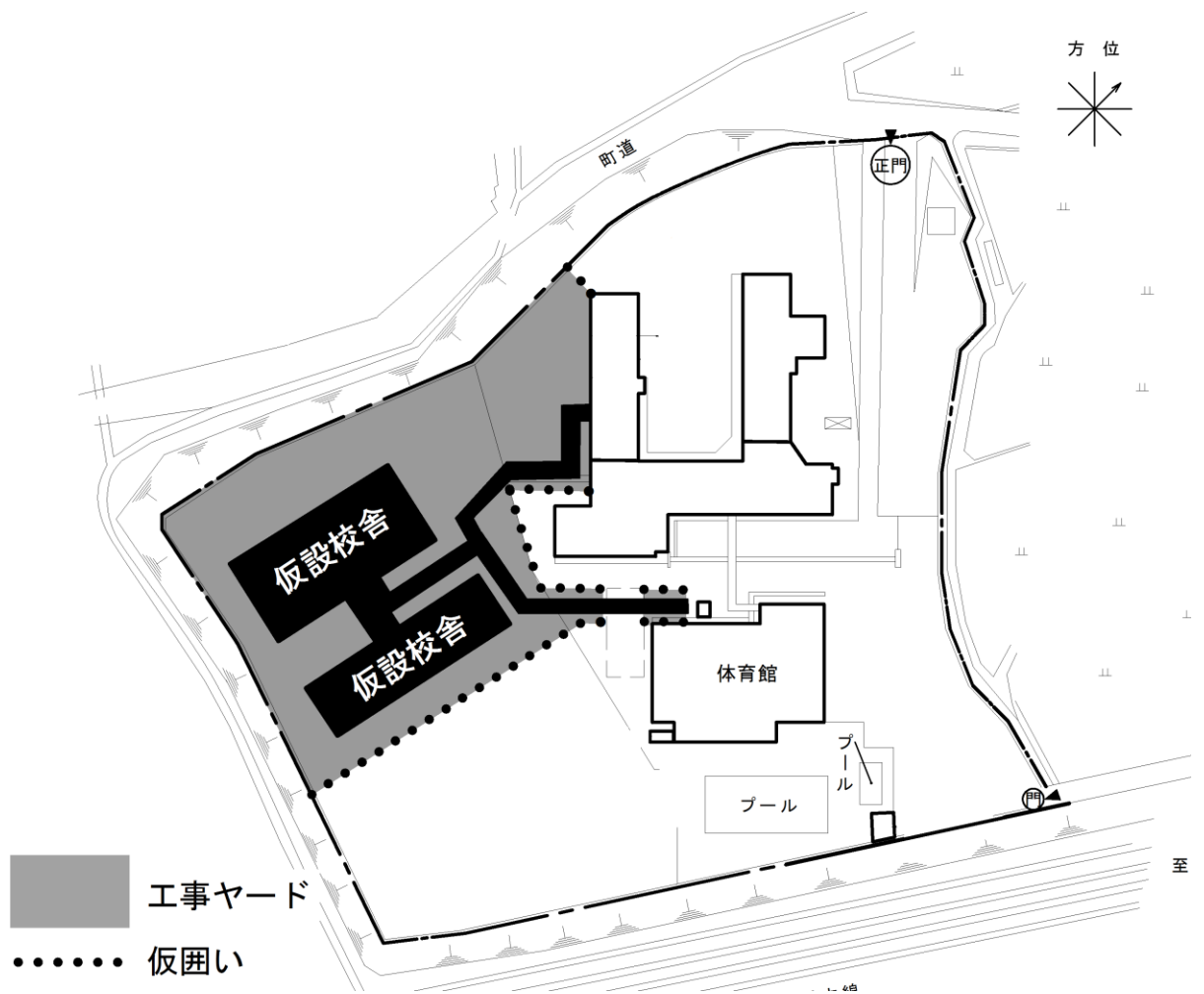
仮設計画図
